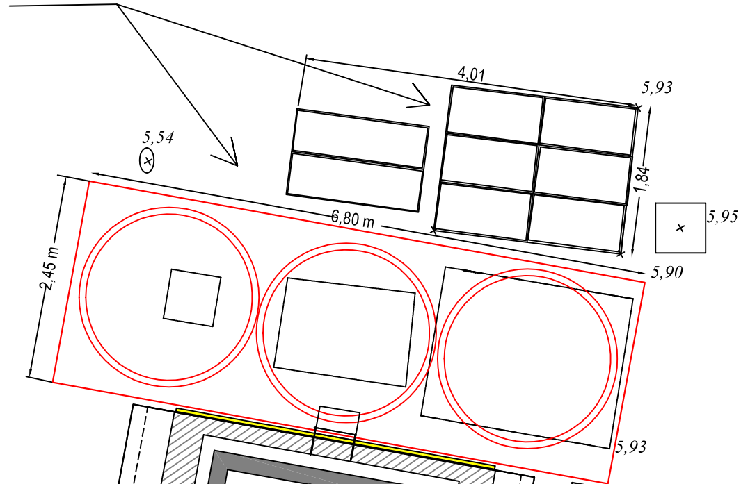
Attuale impianto di sollevamento
