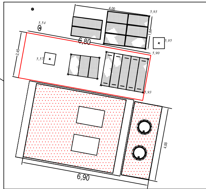
Planimetria a quota strada dell'impianto esistente e di quello in progetto
