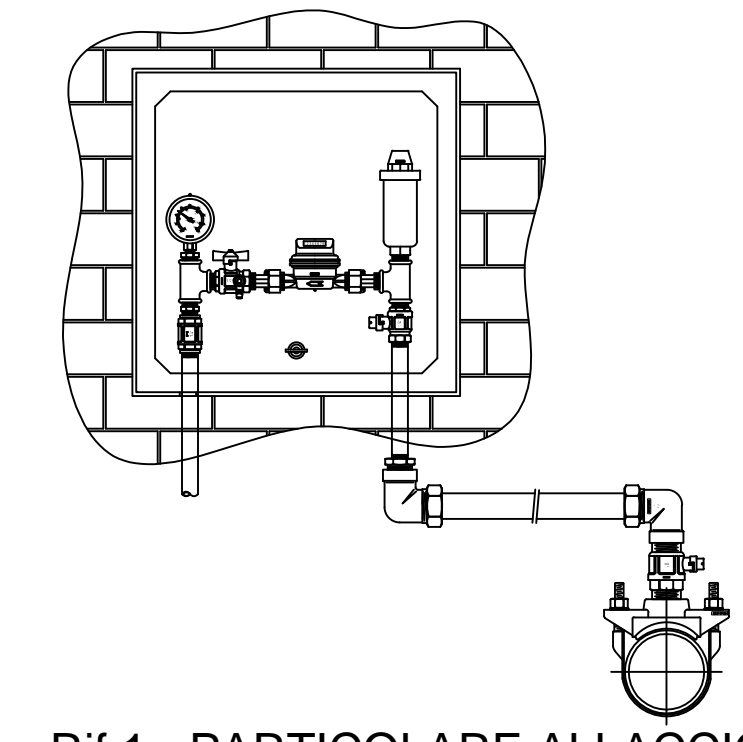
Rif. 1 - PARTICOLARE ALLACCIO CONTATORE IDRICO Scala 1:10
