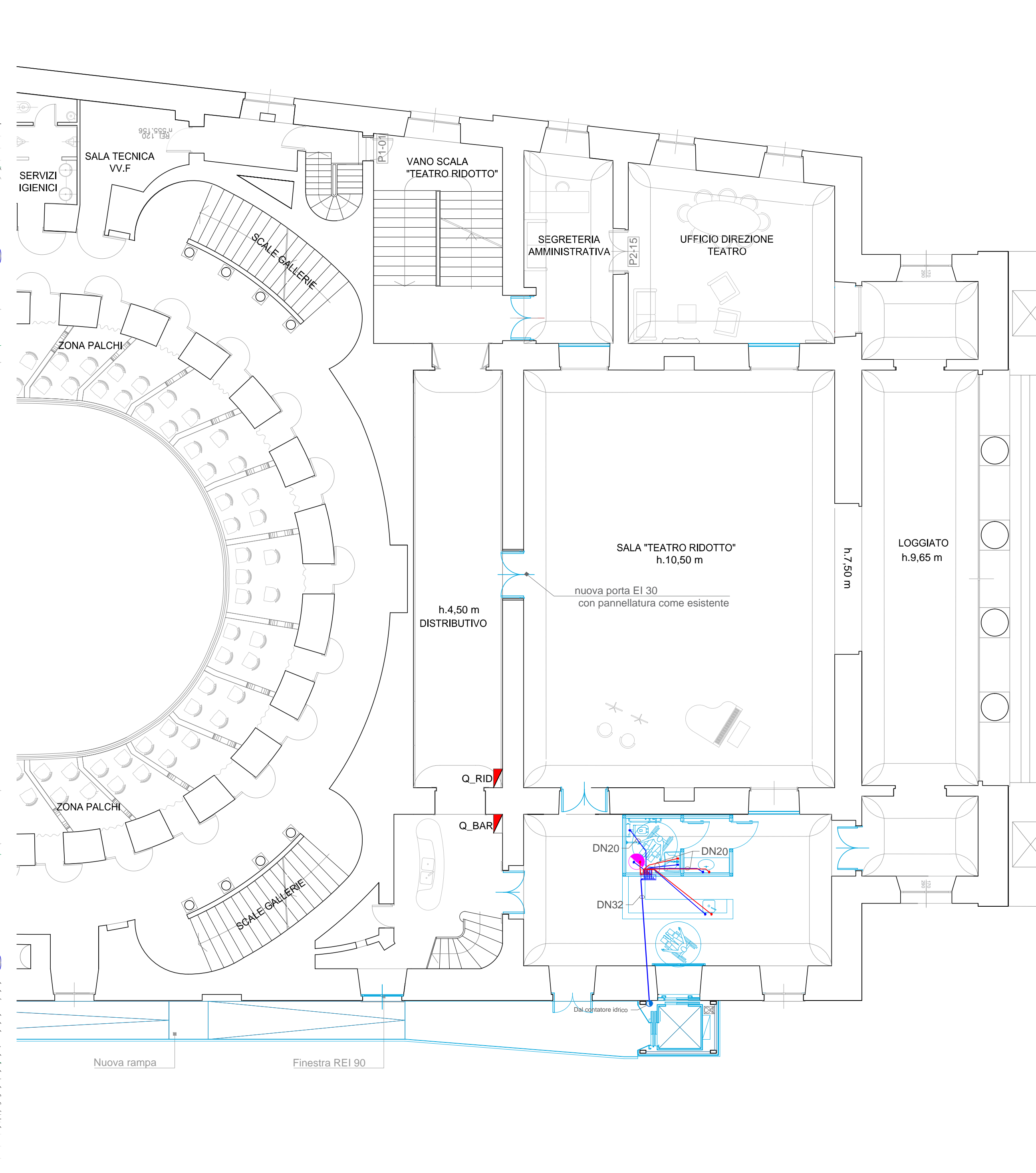
PIANTA PIANO SECONDO Q=XXm
